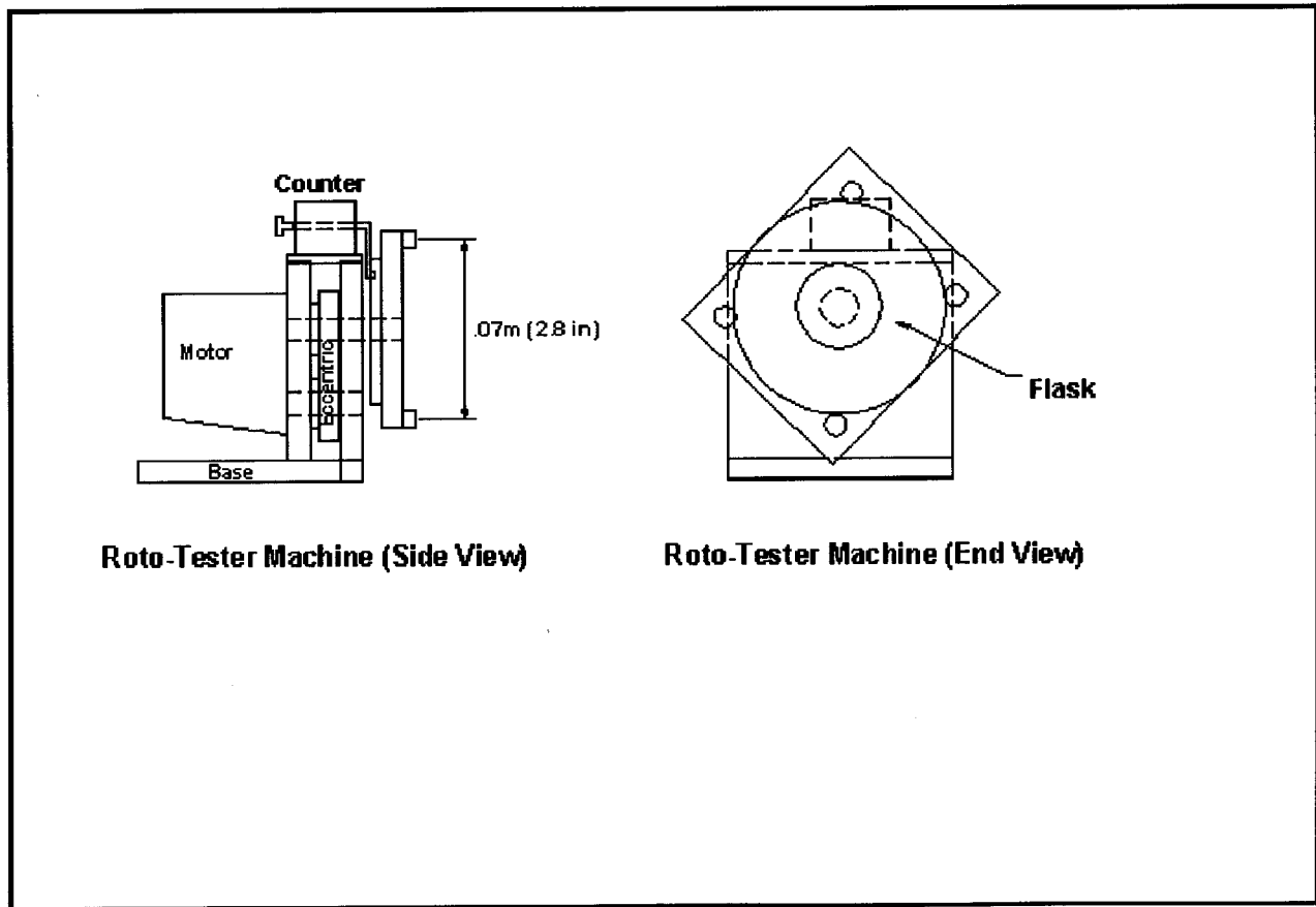
FIG. 2 Roto-Tester
