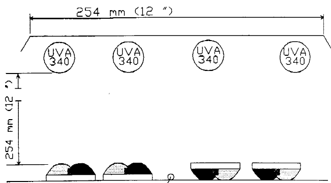
FIG. 2 UV Exposure Apparatus
