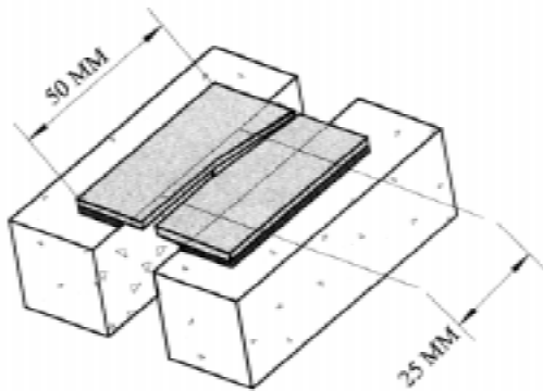
FIG. 6 Tear
