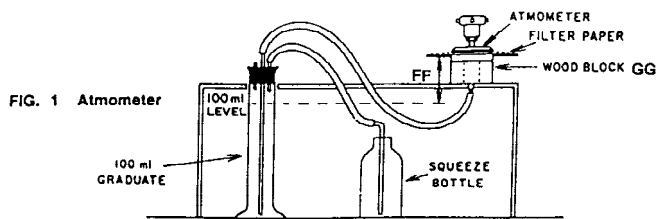
FIG. 2 Atmometer Assembly
