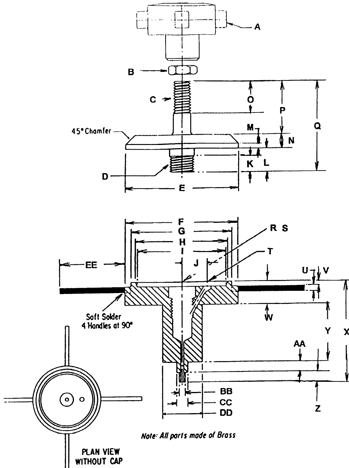
FIG. 1 Atmometer
