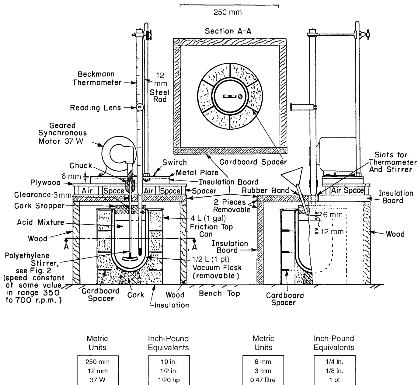
FIG. 1 Calorimeter
