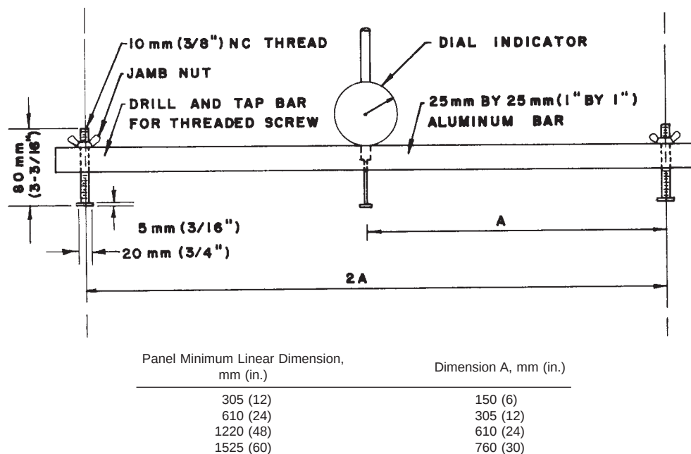
FIG. 2 Sag Bar
