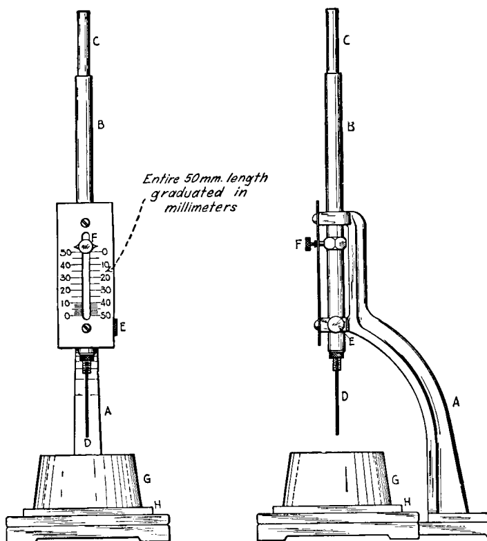
FIG. 3 Vicat Apparatus
